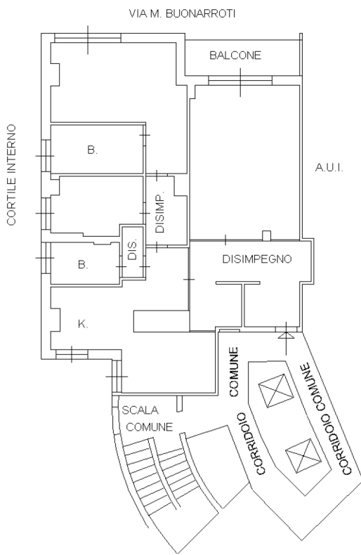
PIANO SECONDO - H. 3.10
